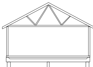
Esempi di incavallature inchiodate
